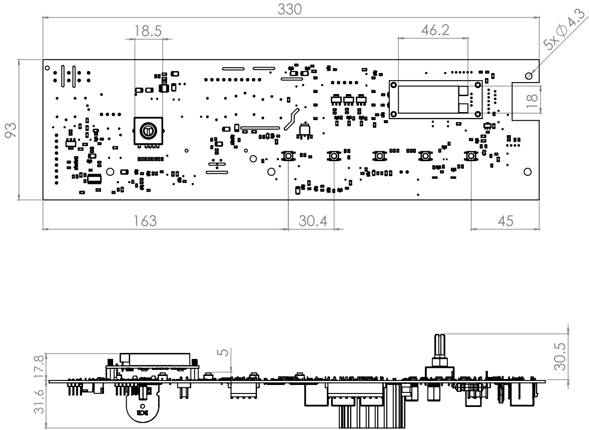
Çamaşır makinesi tahtası GW10 , Laundry Controler
