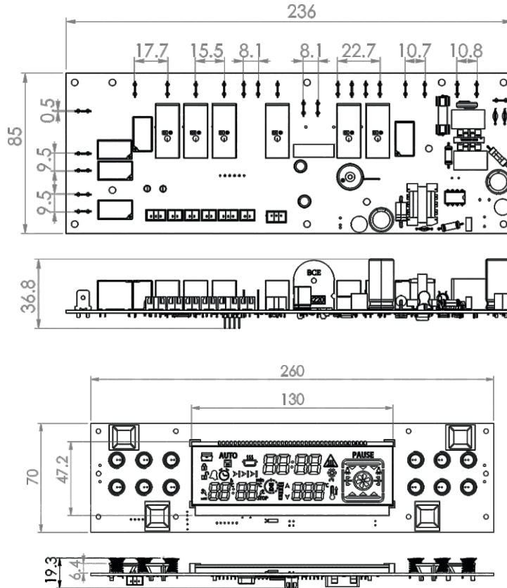
Fırın kontrol panosu 13 işlevi 130P , Electric Oven Controller
